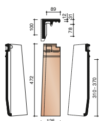
Actua gavl 1/2 stein venstre (1,4 stk/lm)
