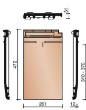
Actua dobbelvalst venstre
