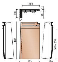
Actua gavl venstre (1,4 stk/lm)
