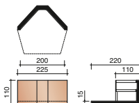
Actua vinkelmøne slutt
