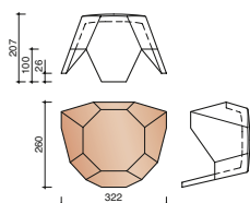
Valmklokke for vinkelmøne 2800
