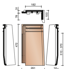
Actua gavl høyre (1,4 stk/lm)
