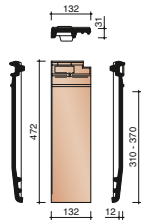
Actua dobbelvalst 1/2 stein venstre
