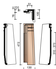
Actua gavl 1/2 stein høyre (1,4 stk/lm)
