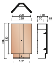
Actua vinkelmøne (3 stk/lm)
