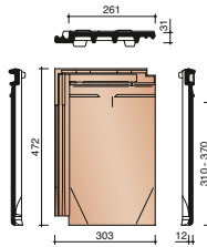
Actua luftstein med gitter
