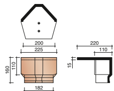
Actua vinkelmøne begynner
